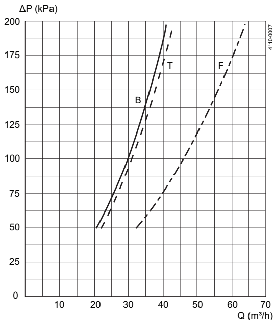
Тип LKRK 94 с 3 мм отверстиями, 51 мм (DN50) трубка: отверстия снизу, отверстия сверху, отверстия везде
