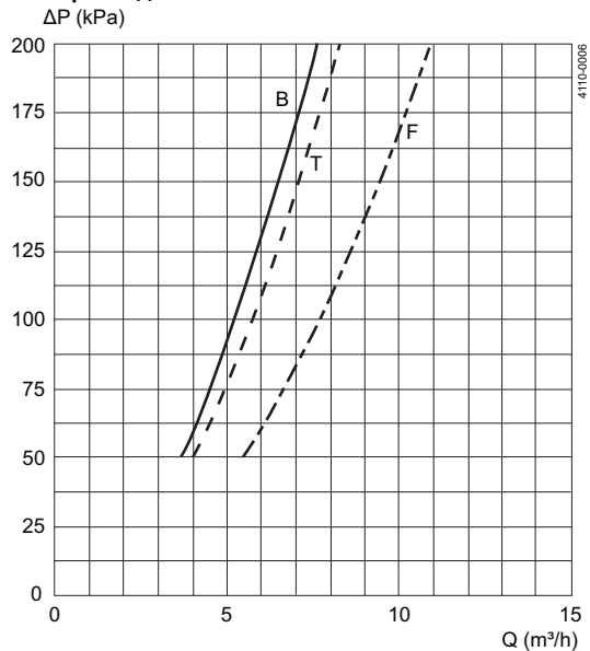
Тип LKRK 64 с 2 мм отверстиями: отверстия снизу, отверстия сверху, отверстия везде
