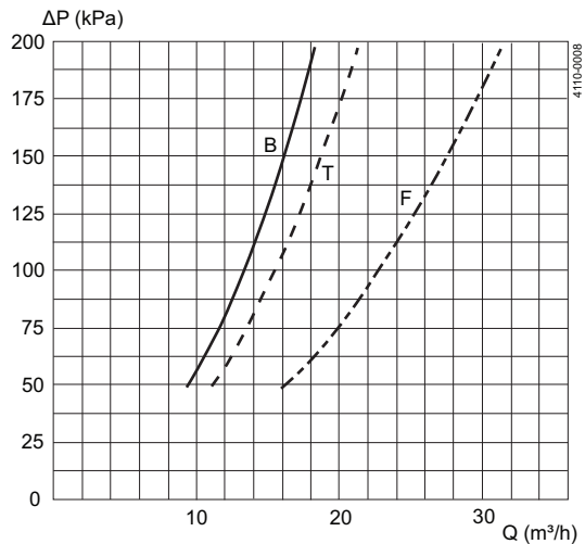
Тип LKRK 94 с 2 мм отверстиями, 51 мм (DN50) трубка: отверстия снизу, отверстия сверху, отверстия везде
